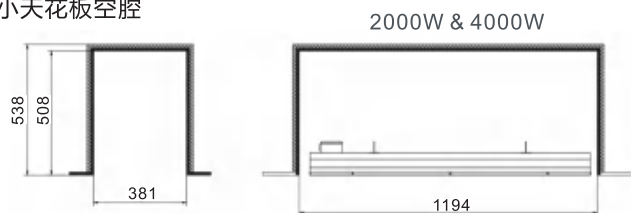
最小天花板空腔
